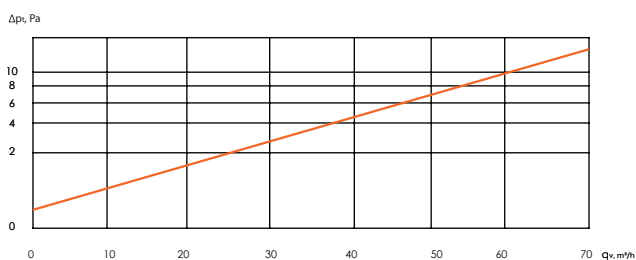
AERO-PRO, SLIM BOX 2x75 (odvod vzduchu)
