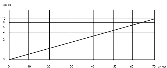
AERO-PRO, SLIM BOX 2x75 (přívod vzduchu)
